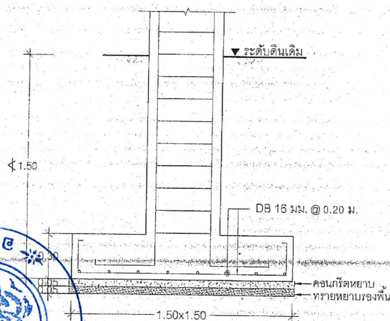
แบบแปลน F1 Scale 1:25
